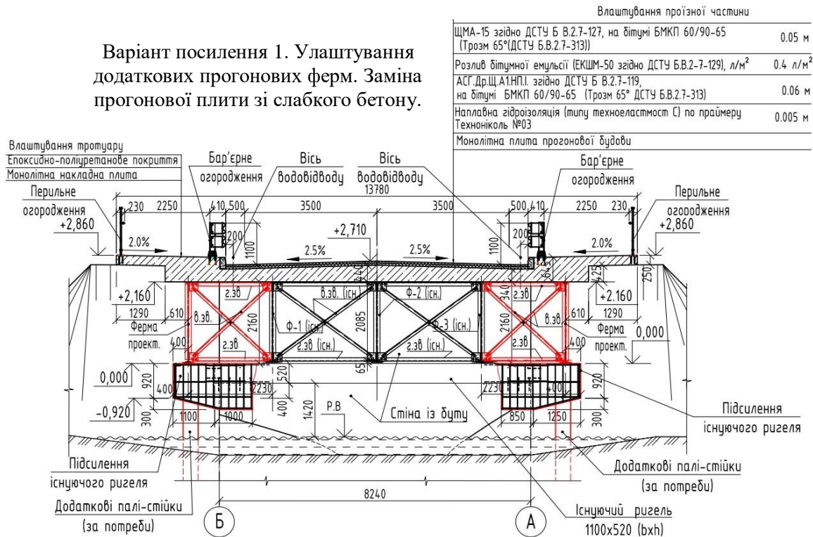
Рисунок 4 – Принципова схема посилення і розширення прогонової будови мосту по варіанту 1 улаштуванням двох додаткових металевих ферм. Червоним виділено нові металлоконструкції.
