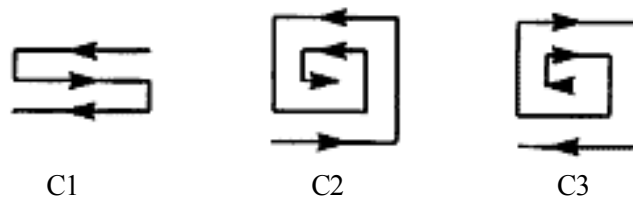
Рисунок 2 – Порядок забивки паль у групі
